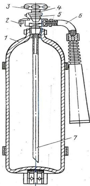
Р и с. 21. Углекислотный огнетушитель ОУ-5: 1 – баллон; 2 – предохранитель; 3 – маховичок вентиля-запора; 4 – металлическая пломба; 5 – вентиль; 6 – поворотный механизм с раструбом; 7 – сифонная трубка.
